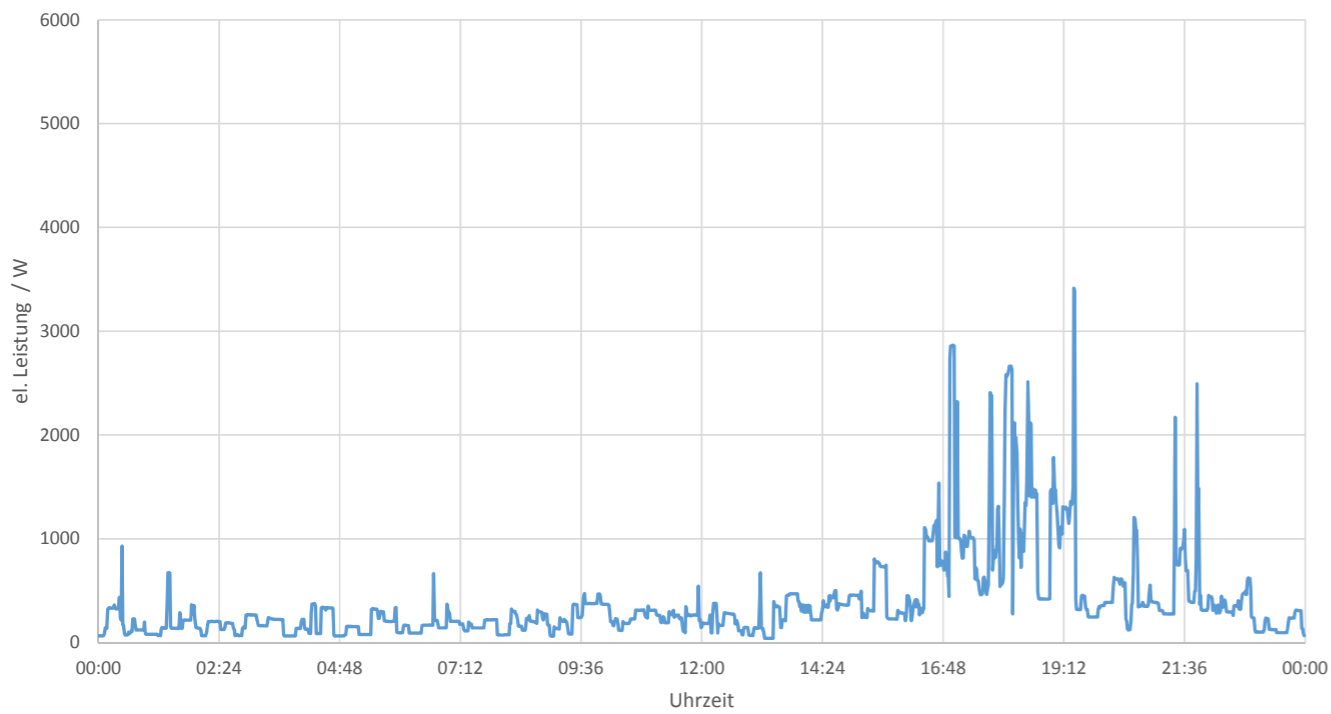
Lastprofil - 20.06.2010
